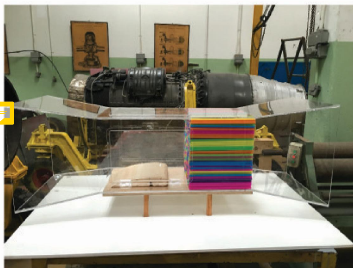
Δράση 3: Κατασκευή εκπαιδευτικού μοντέλου αεροσήραγγας
